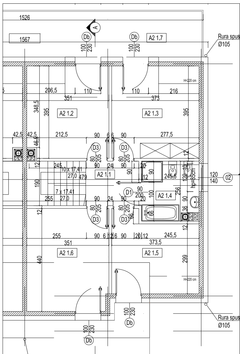
RZUT PIĘTRA
