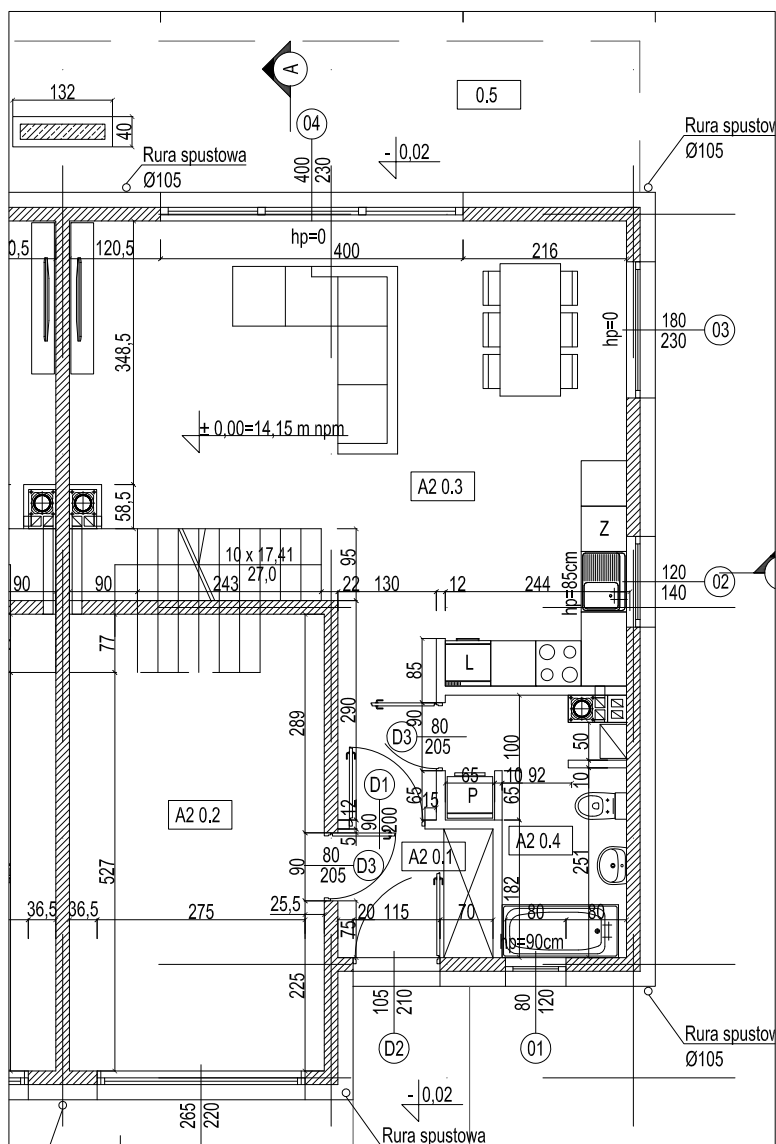
RZUT PARTERU
