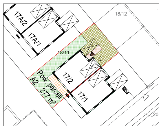
PLAN SYTUACYJNY
